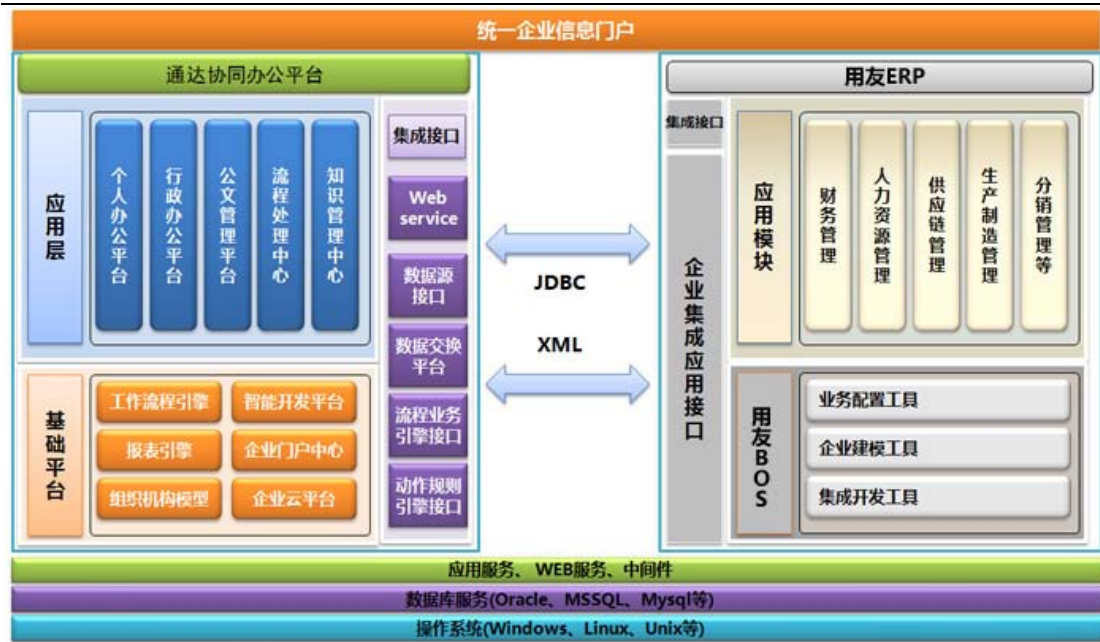
图 1 通达 OA 和用友 ERP 集成系统构架图
